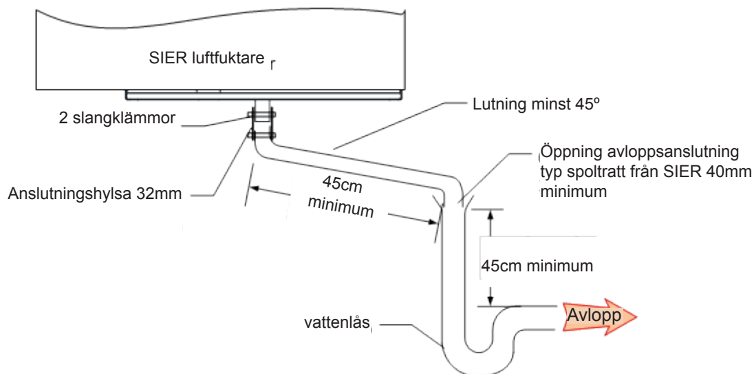
Figur 12 – anslutning av tömning och dränering avloppsvatten
