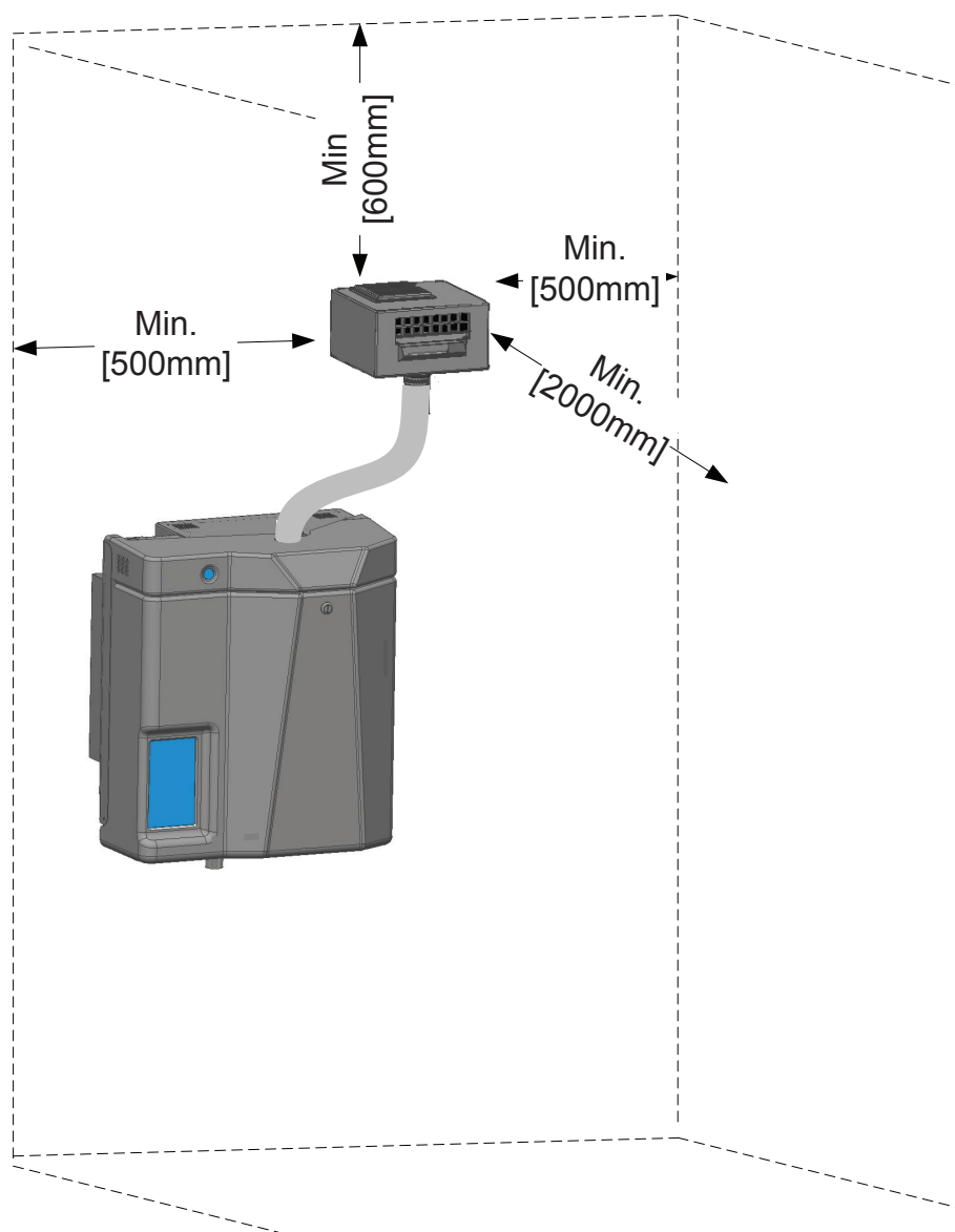
Figur 7 – minimikrav för fläkt SBL -M -S
