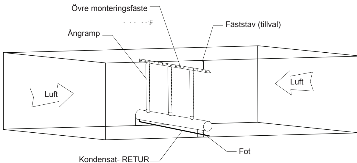
Figur 26 – installation av steamOsorb multiramp
