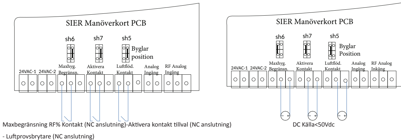
Figur 29 – anslutning av styrsignal
