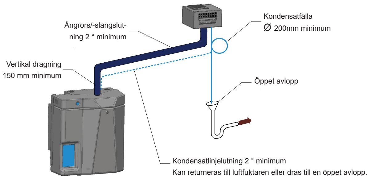
Figur 15 – ång- och kondensledning för separat fläktdeinstallation
